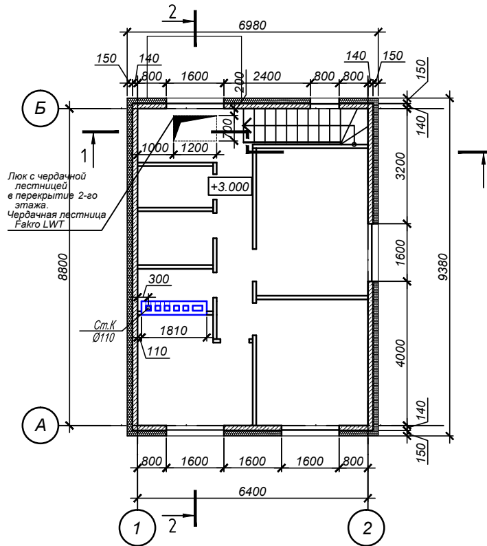
План 2 этажа
