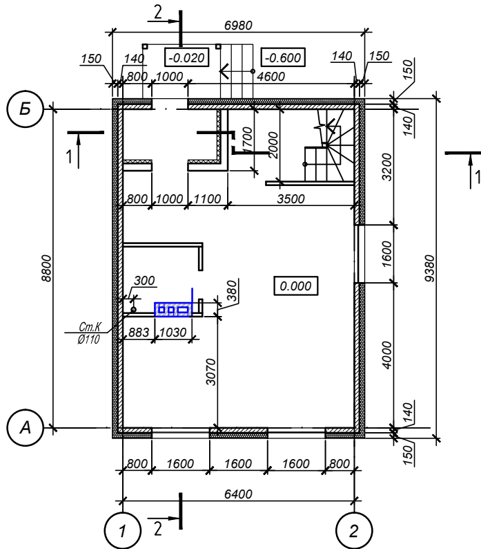
План 1 этажа
